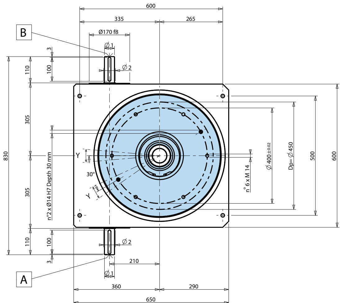
Rotating element • Elemento rotante • Drehelement • Élément tournant • Elemento de giro
